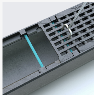
Schraublose Verriegelung
