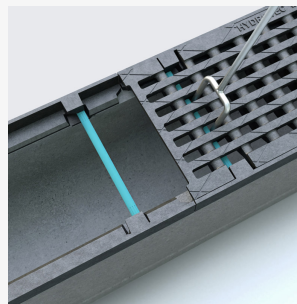
Schraublose Verriegelung
