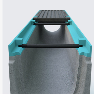
Kantenschutz
